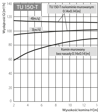
Wykres wydajności obrotowych nasad kominowych TULIPAN dla kominu mурowanego dla dwóch prędkości wiatru 3 i 4 [m/s].
