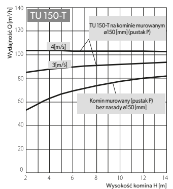
Wykres wydajności obrotowych nasad kominowych TULIPAN dla kominu mурowanego (pustak typu P) dla dwóch prędkości wiatru 3 i 4 [m/s].
